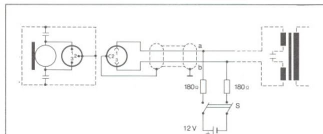
Symmetrische Tonaderspeisung nach DIN 45 595
