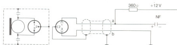
Alimentation symétrique par conducteurs de modulation selon DIN 45 595
