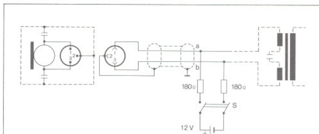
Alimentation symétrique par conducteurs de modulation selon DIN 45 595
