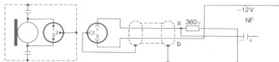
Alimentation asymétrique conducteurs de modulation
