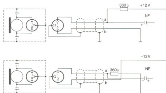
Unsymmetrische Tonaderspeisung
