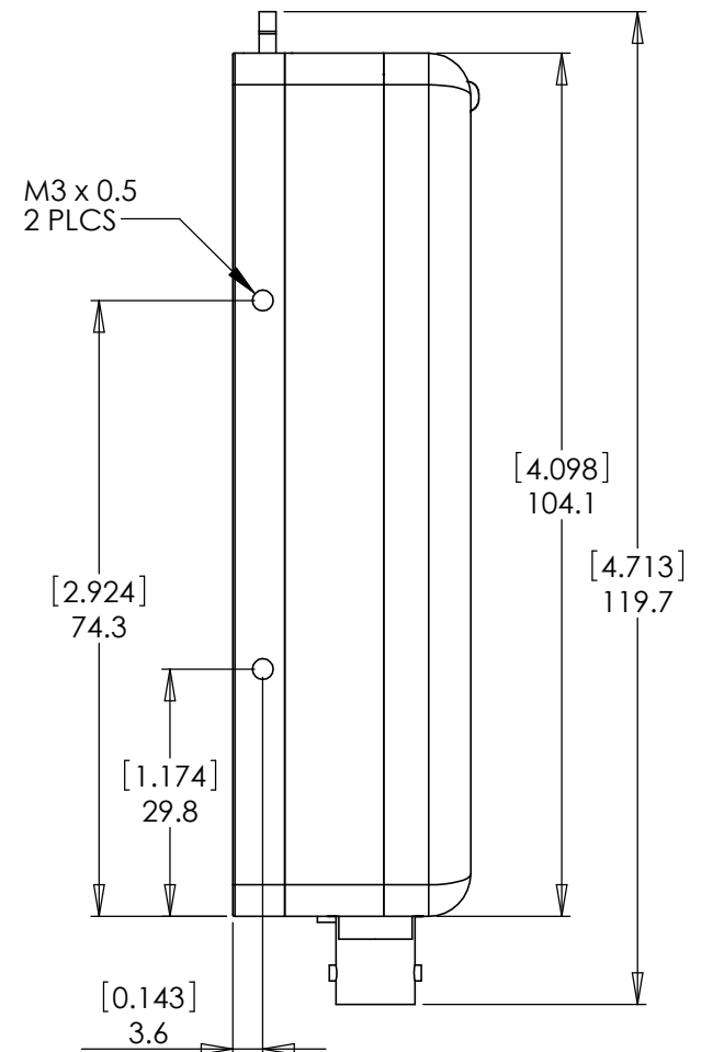
LEFT
